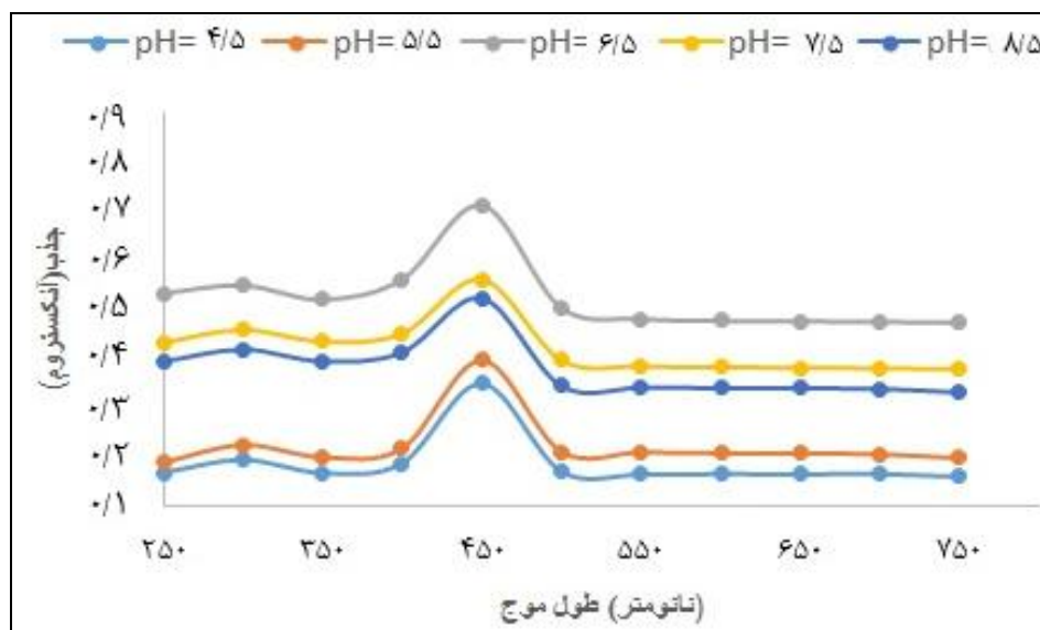
نمودار ۱. طیف اسپکتروفتومتری فرابنفش - مری محلول حاوی نانوذرات نقره سنتز شده در pH های مختلف
