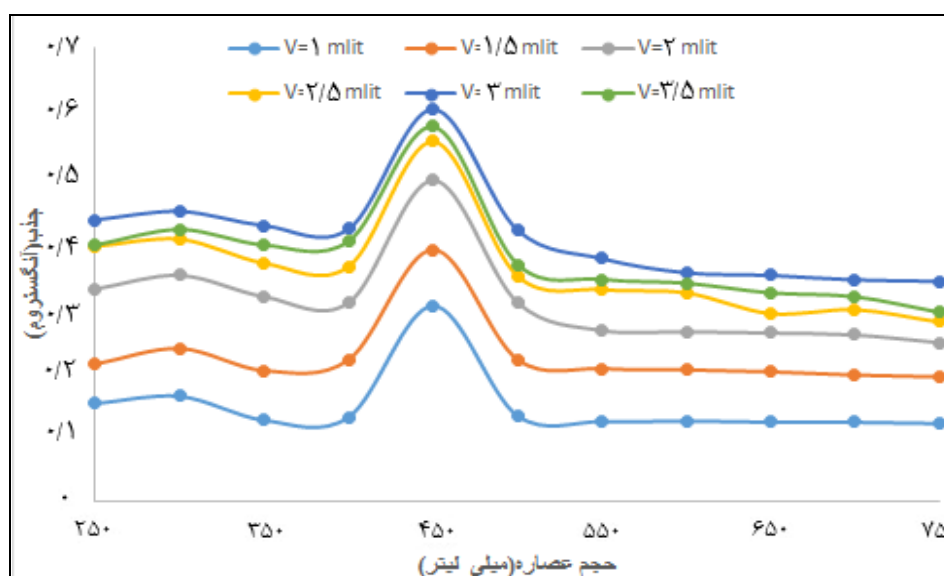
نمودار ۲. طیف اسپکتروفتومتری فرابنفش - مری محلول حاوی نانوذرات نقره سنتز شده در حجم های مختلف عصاره
